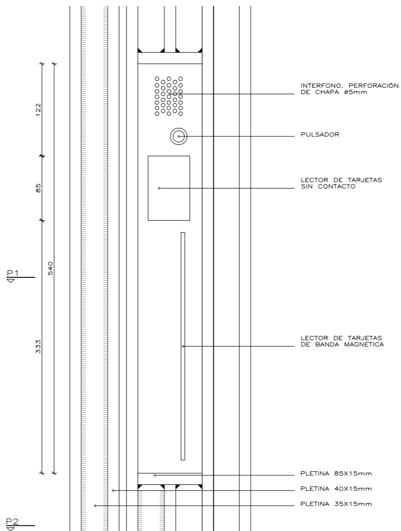
ALZADO EXTERIOR
