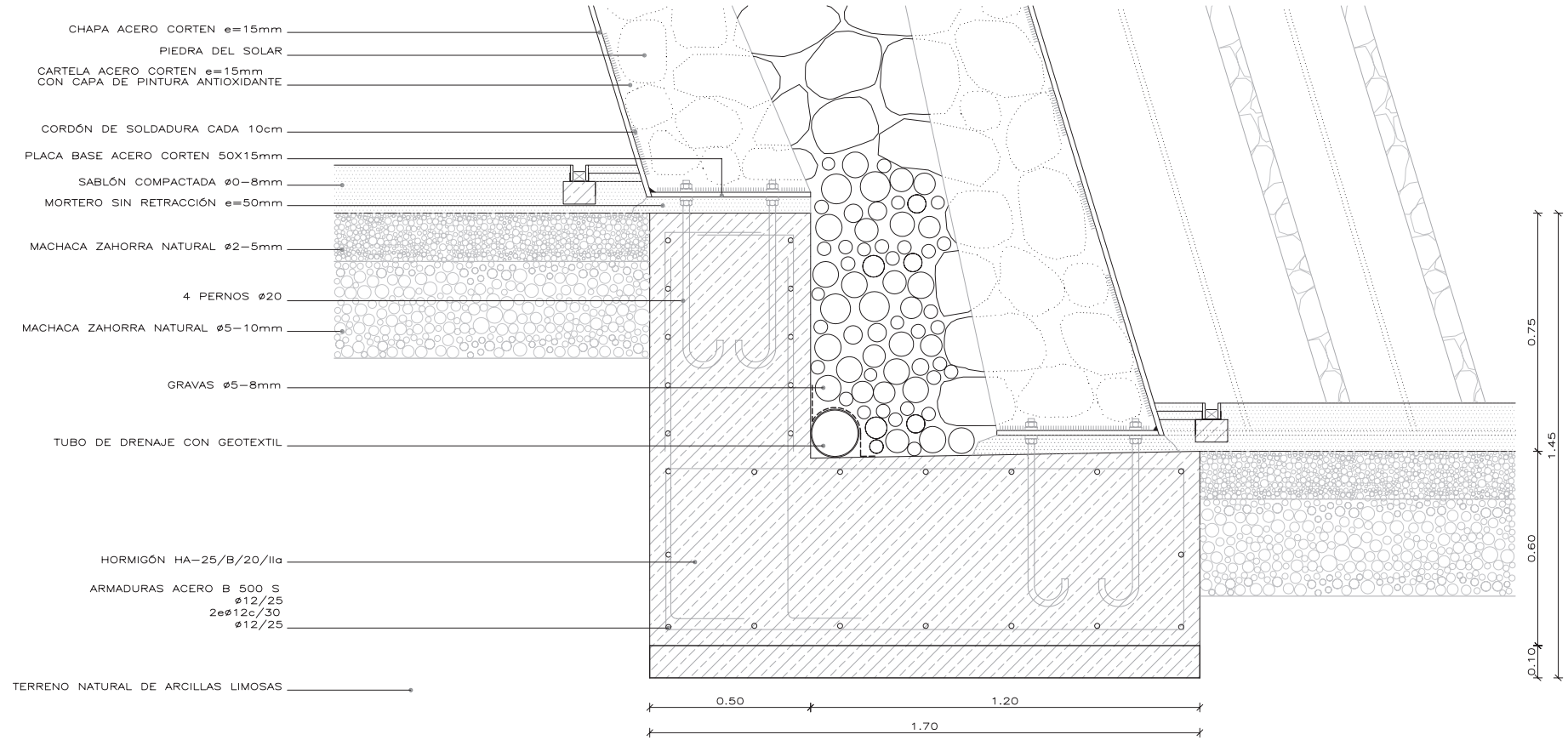
D1-DETALLE SECCIÓN TRANSVERSAL 0 0.4M
