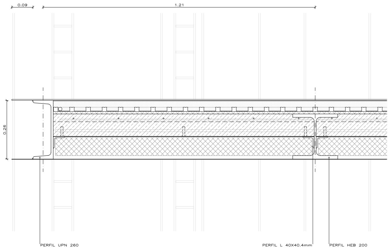
DETALLE SECCION LONGITUDINAL 0 0,2M
