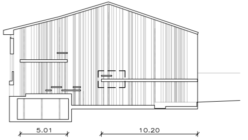
SECCION LONGITUDINAL 0 8M
