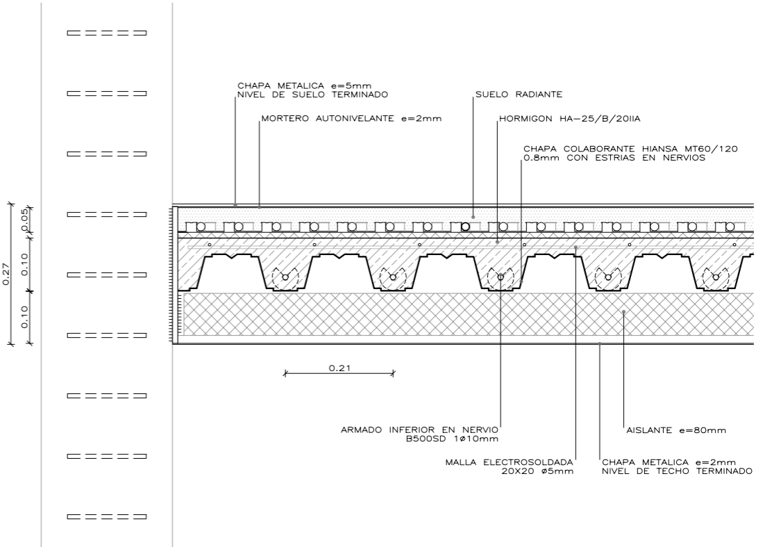
SECCION LONGITUDINAL 0 8M
