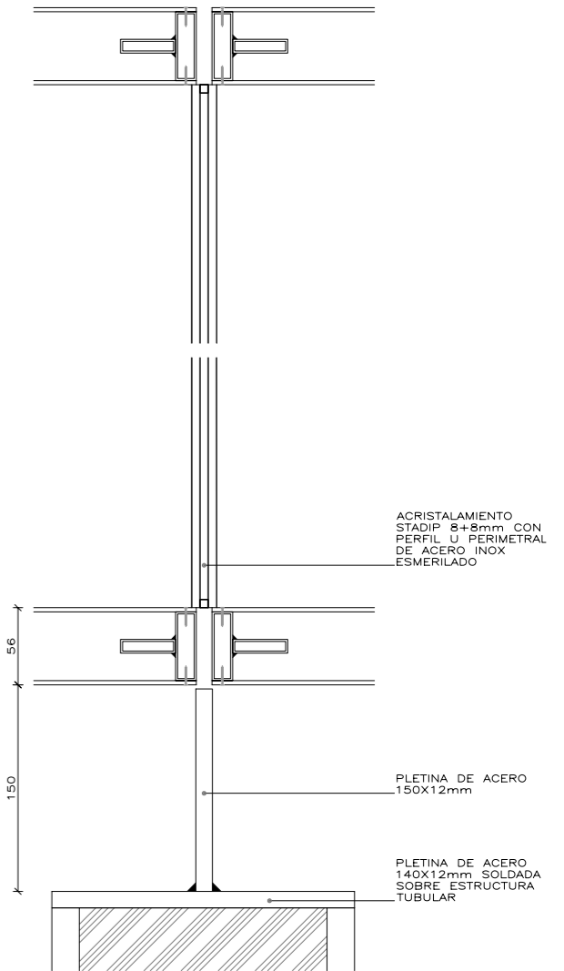
DETALLE PLANTA 0 0,04M
