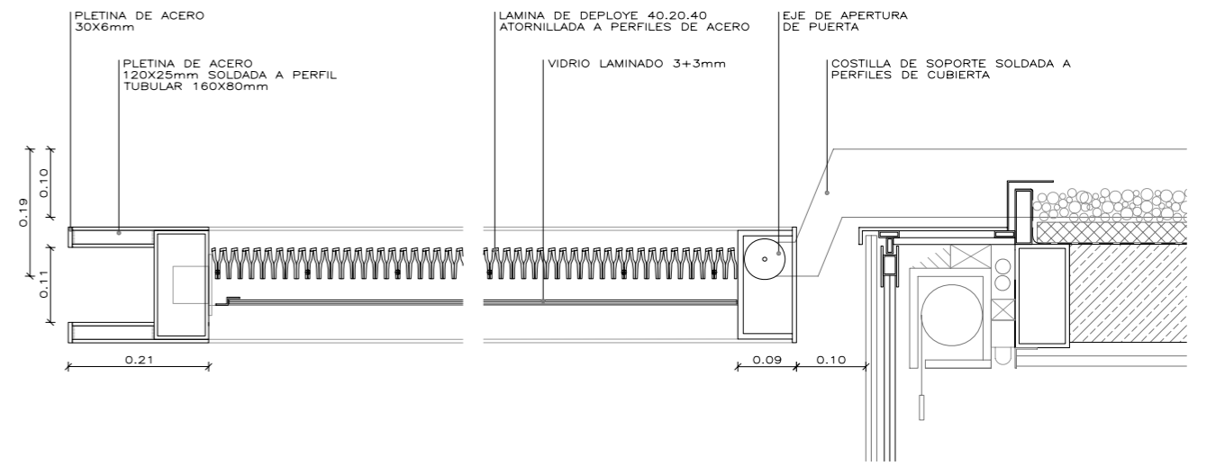
D1 D2 DETALLE SECCION 0 0,2M
