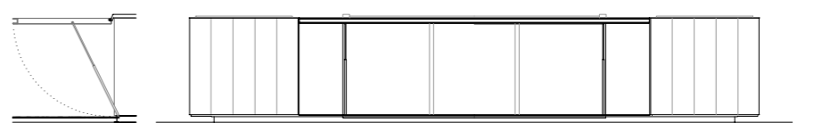
ALZADO Y SECCIÓN PORCHE HIDRÁULICO ABIERTO 0 4M
