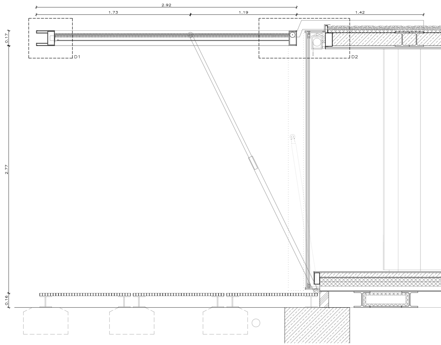
DETALLE PORCHE SECCIÓN VERTICAL 0 0,5M
