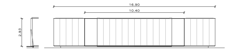
ALZADO Y SECCIÓN PORCHE HIDRÁULICO CERRADO 0 4M
