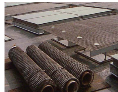
Cubierta plana de malla de acero - Dominique Perrault. Velódromo y piscina olímpica en Berlín © Hisao Suzuki
