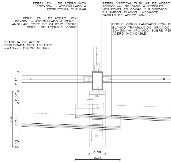
DETALLE PLANTA 0 0,2M
