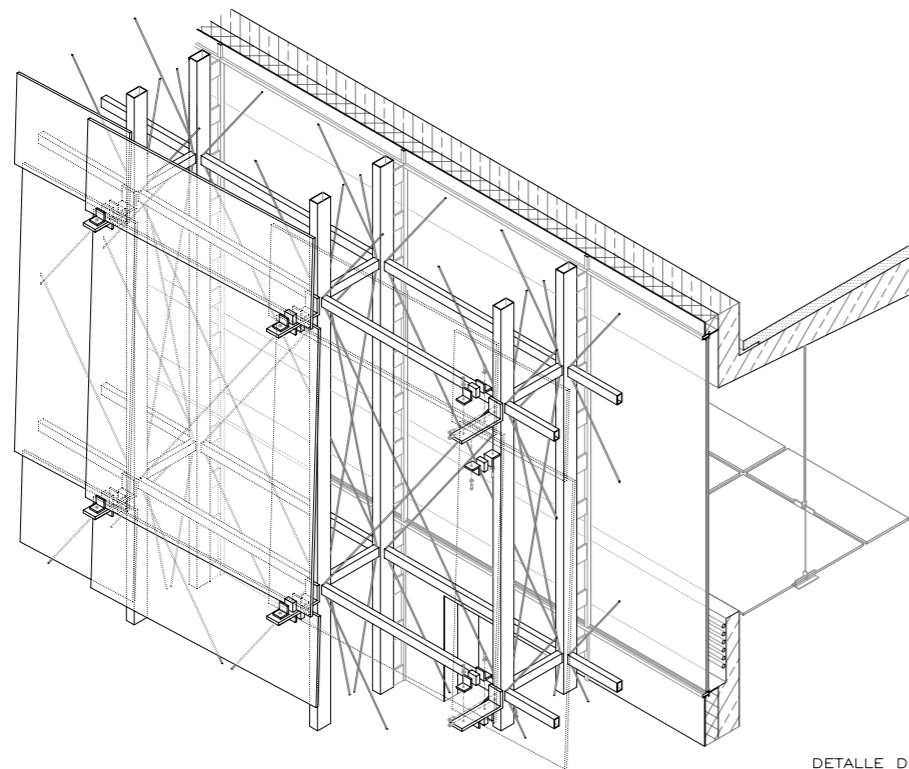
DETALLE SECCIÓN
