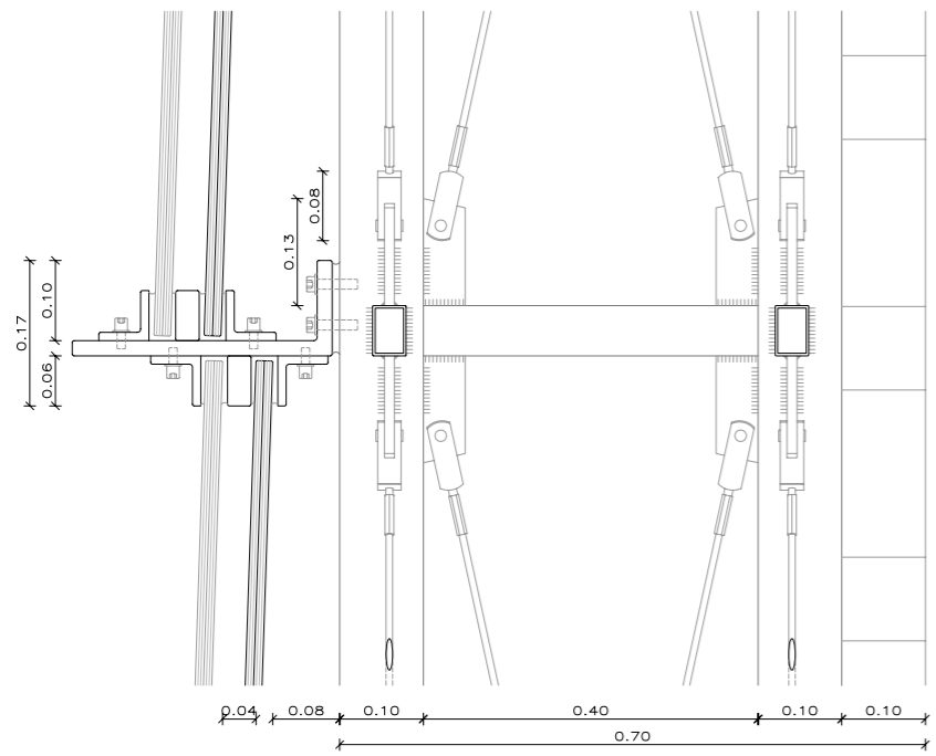
DETALLE SECCIÓN
