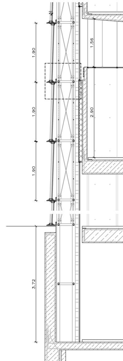
SECCIÓN TRANSVERSAL
