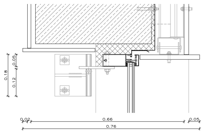
D1 PLANTA EN PILAR
