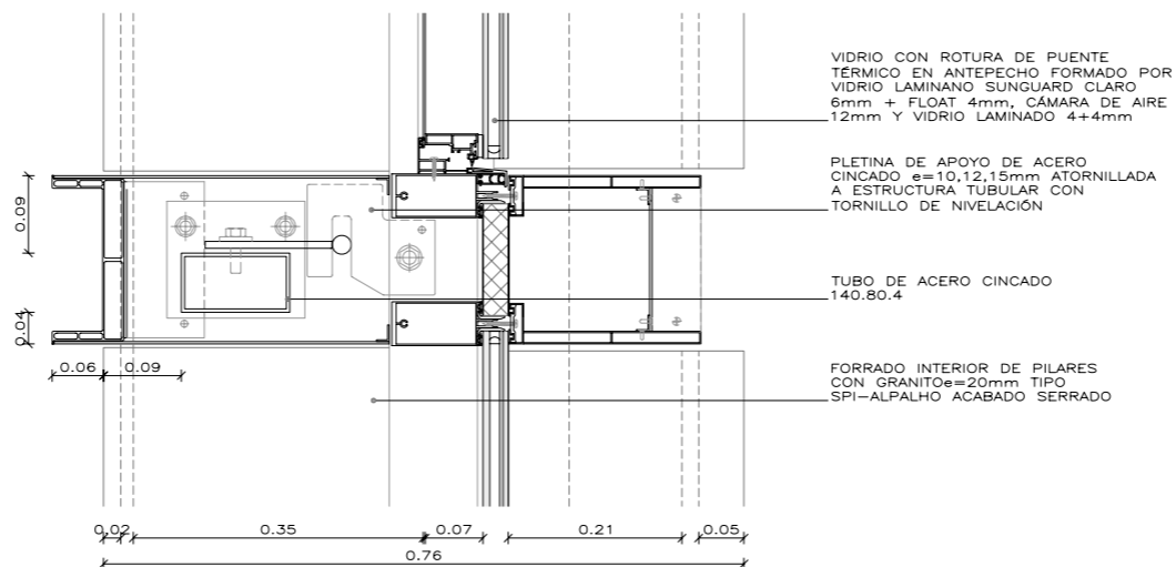
D3 SECCIÓN A MEDIA ALTURA 0 0,2M
