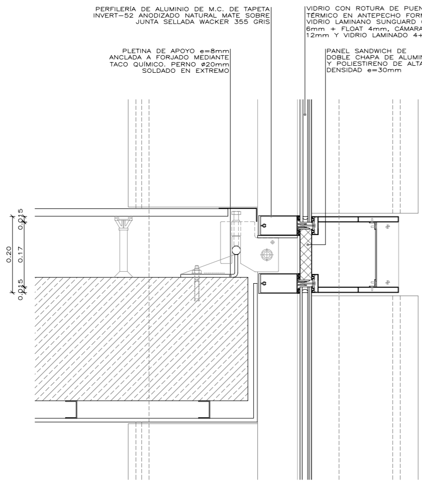
D1 SECCIÓN EN FORJADO
