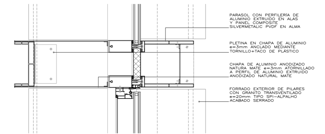
D2 SECCIÓN A MEDIA ALTURA EN PILAR
