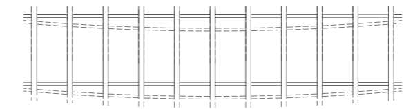
ESQUEMA DE DEFORMACION VIGA VIEREENDEL
