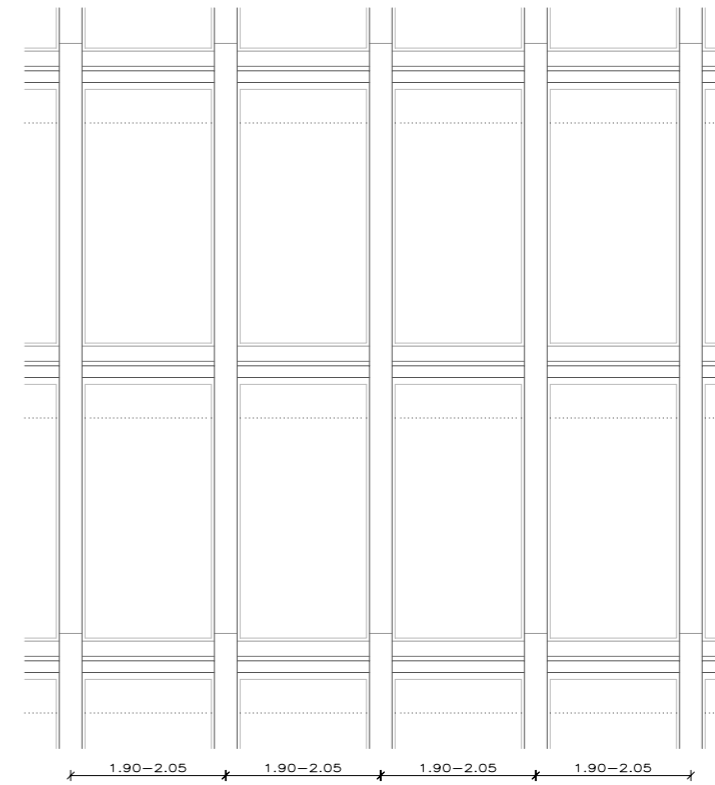
ALZADO GENERAL
