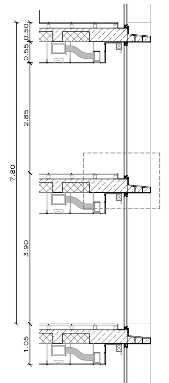
SECCION 0 2M
